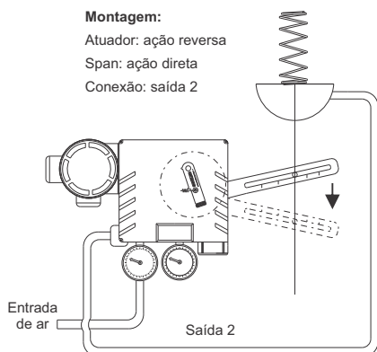
Posição do SPAN
