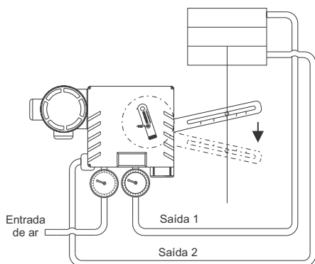
Posição do SPAN
