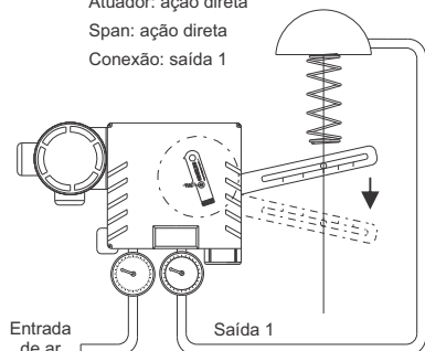
Posição do SPAN
