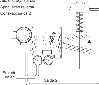
Posição do SPAN
