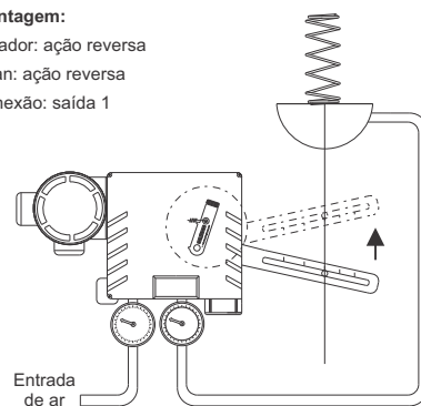
Posição do SPAN
