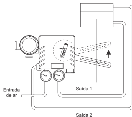
Posição do SPAN
